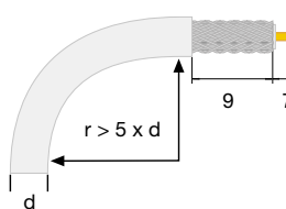
Рис 1: Радиусы изгиба и длина изоляции
