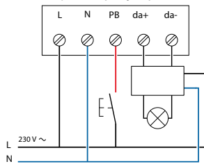
Рис 6: Подсоединение инфракрасного датчика присутствия
