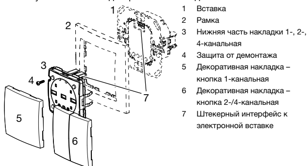
Рис 1: Монтаж на примере радиопоины KNX
