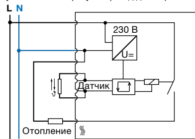
Рис 6: Схема подключения Регулятор температуры, включаемый по времени, с замыкаемым контактом и центральной панелью
