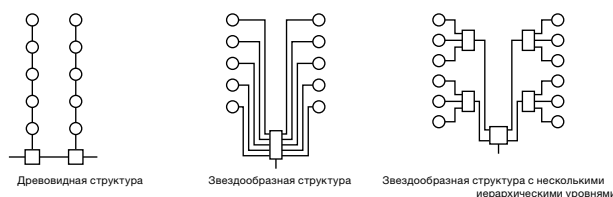
Рис 1: Структуры кабельных соединений
