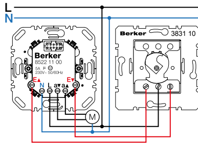
Рис 3: Единичное управление с дополнительным устройством «Жалюзи́нная замочная кнопка 1-полюсная» для профильного полуцилиндра
