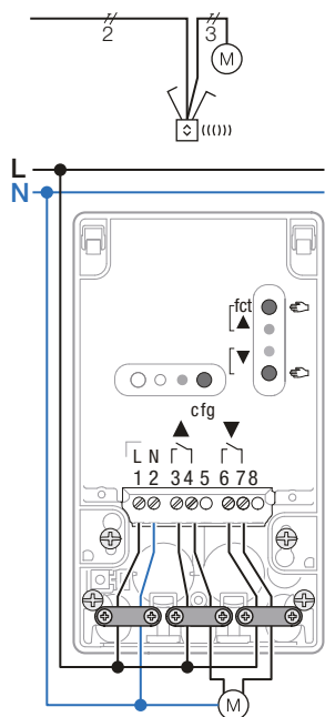
Рис 1: Управление двигателем
