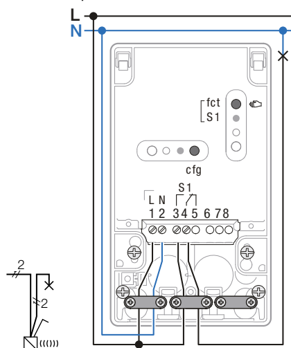
Рис 1: Переключение лампы
