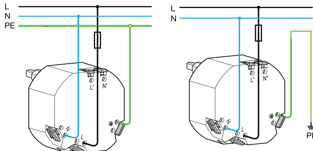
Рис 3: Подсоединение в сети TN-S/TT
