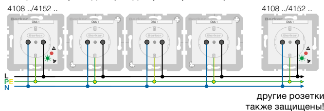
Рис 3: Установка в комбинации с розетками SCHUKO
