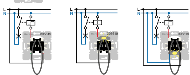
Рис 5: Шнуровая кнопка, переключающий контакт/шнуровая кнопка с подсветкой: ограничивайте количество параллельно подключенных кнопок или проводите нейтральный провод/шнуровая кнопка с постоянной подсветкой: неограниченное количество подключаемых параллельно кнопок, необходимо проведение нейтрального провода/контрольное выключение
