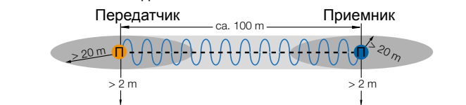
Рис 1: Расстояния до источников помех в свободном поле
