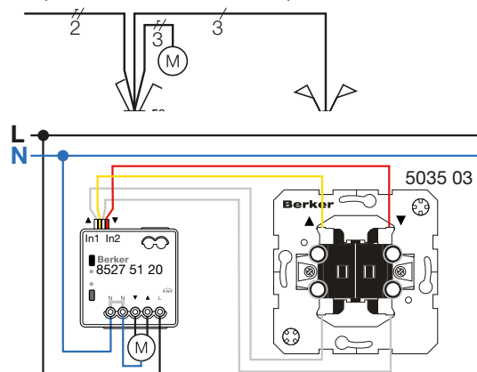
Рис 2: Управление двигателем
