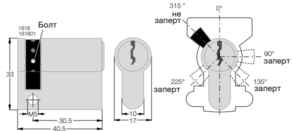
Рис 4: Профильный полуцилиндр [№ для заказа 1818, 1818 01]
